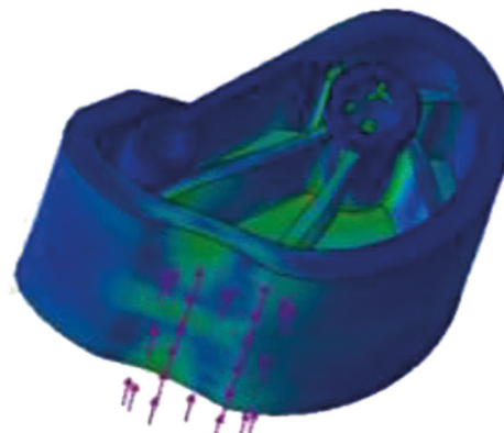
„Tragfix“ Backen
