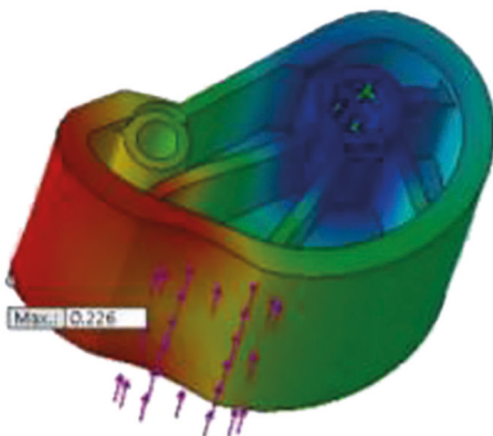
Herkömmliche Backen
